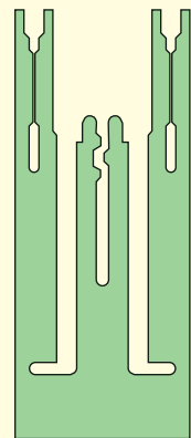
UCS-CM 接続タイプ
